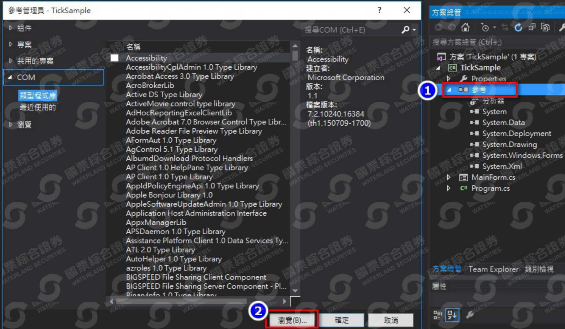
Visual Studio 開發環境畫面
